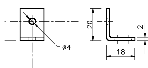
STAFFE DI FISSAGGIO TIPO "S2" (ACCESSORIO) COD. 1210128 "S2" TYPE MOUNTING BRACKETS (OPTIONAL) COD. 1210128
