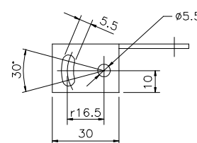
STAFFE DI FISSAGGIO TIPO "S1" (ACCESSORIO) COD. 1210129 "S1" TYPE MOUNTING BRACKETS (OPTIONAL) COD. 1210129
