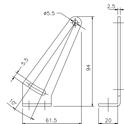
STAFFE DI FISSAGGIO TIPO "S2" (ACCESSORIO) COD. 1210128 "S2" TYPE MOUNTING BRACKETS (OPTIONAL) COD. 1210128
